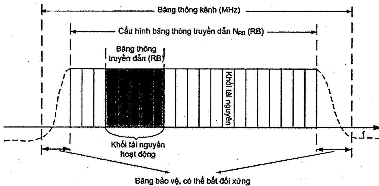
Hình 1 - Bảng thông kênh và cấu hình bảng thông truyền dẫn đối với một sóng mang
