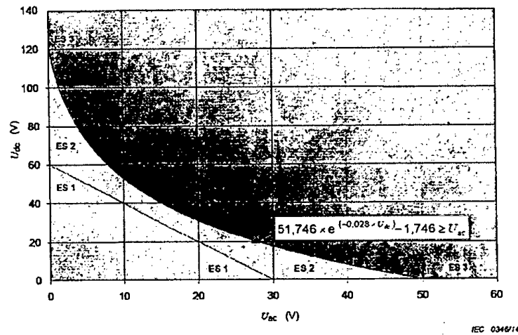
[Hình 23] - Các giá trị cực đại cho kết hợp điện áp a.c và điện áp d.c
